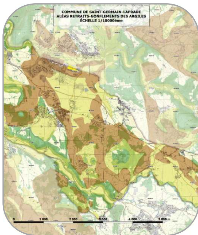
Carte des zones à aléa retrait-gonflement des argiles (Source : IRMa, juillet 2022)
